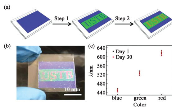
图 3 (a)多色模板的制作方法。第一步:在蓝相薄膜上打印长方形绿色背景色,用 16 V 电压;第二步:在蓝相薄膜上打印红色“USTB”字样,用 24 V 电压;(b) 注射-打印多色模板的照片(标尺:10 mm);(c) 第 1 天和 30 天后模板上不同颜色的区域对应的波长 [76] 。
