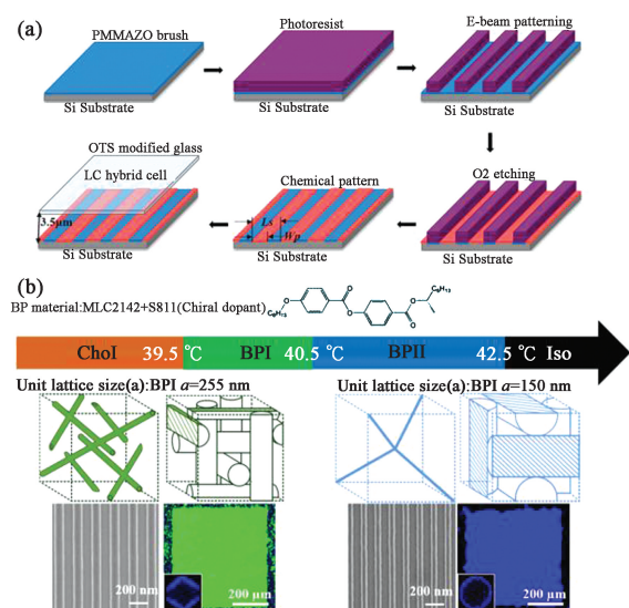
图 2 (a)PMMAZO 梳状分子层取向特性,制备纳米或微米条纹结构的制作步骤示意图,另一面采用垂直锚定的玻璃;(b)升温形成胆甾相、蓝相 I、蓝相 II 和各向同性相,不同周期的条纹模板用来形成单晶蓝相 I (110)和蓝相 II(100),分别对应 40.1 °C 和 41.7 °C,左下角插图为相应的 Kossel 图像 [75] 。
